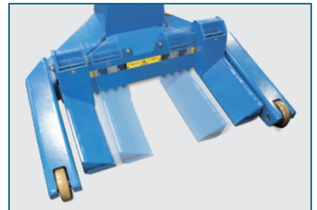
Carrello a forche regolabili per diametro ruote da 500 mm a 1200 mm. Adjustable forks for wheels from 500 to 1200 mm in diameter. Vertellbaren Radgreifern auf Radgrößen von 500 mm bis 1200 mm. Chariot avec fourches réglables pour diamètre de roue de 500 mm à 1200 mm. Carros regulables para ruedas de diametro 500 mm a 1200 mm.
