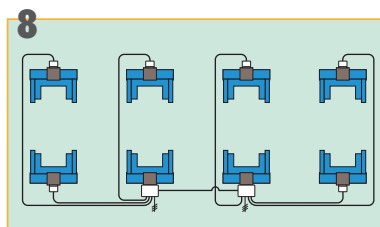
Attacchi per forche Fork supports Gabelunterstützung Supports de fourche Soportes de horquilla
